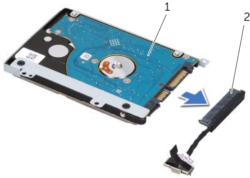
1 zostava pevného disku 2 premost'ovač
